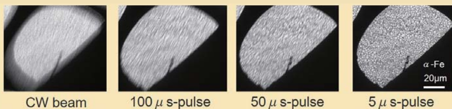
1kHzで揺れ動く試料にパルス電子線をもちいた場合のTEM像
