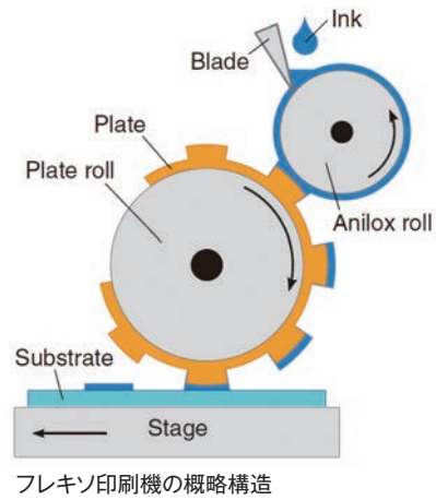
フレキシ印刷機の概略構造
