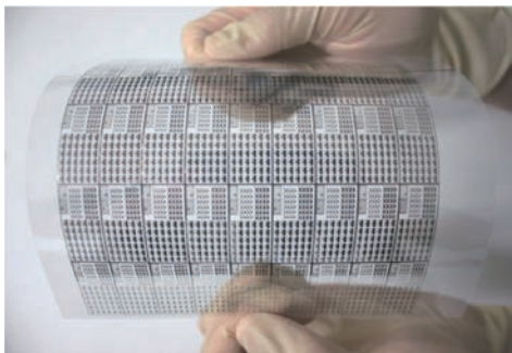
15×15cm 2 の透明フレキシブルプラスチックフィルム上に配列印刷されたCNT TFT(=Thin Film Transistor)
