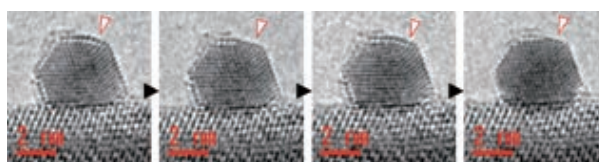
図1 99%Ne-1%NOガス中のZrO 2 担持Rhナノ粒子の表面構造変化(500°C)の電子顕微鏡像
