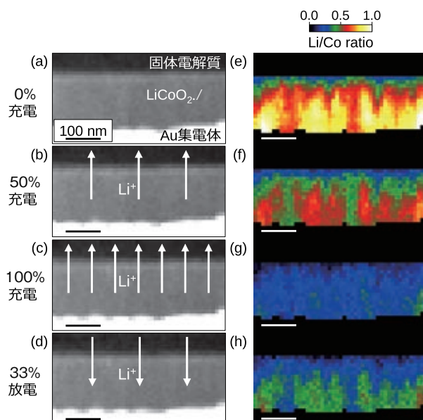
図1: 充放電中における \text{LiCoO}_2 正極内部のLiイオン濃度分布の変化。(a)~(d) 固体電解質/ \text{LiCoO}_2 正極/Au集電体近傍の断面STEM像。それぞれ、0%充電(充電前)、50%充電、100%充電、33%放電時のSTEM像を示す。(e)~(h) EELSと高度画像解析を用いてマッピングされた同一箇所のLi分布。固体電解質との界面近傍で、イオン濃度が低いことがわかる。また、充電が進むにつれて、 \text{LiCoO}_2 正極からLiイオンが脱離し、濃度が低下していることがわかる。放電時には、Liイオンが戻ってくるため、Au集電体に近いところからイオン濃度が高くなっていることがわかる。
