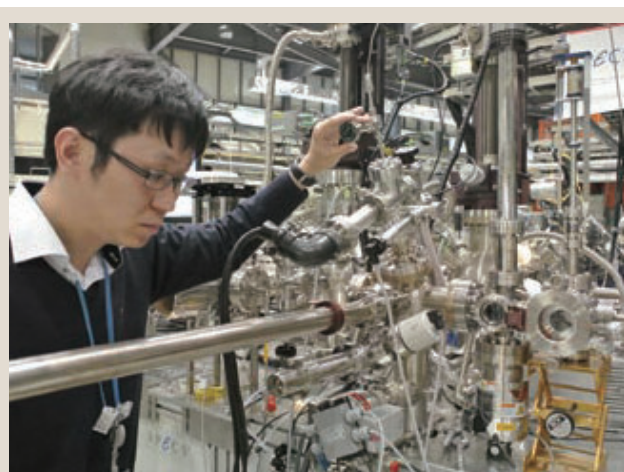
あいちSRセンターの軟X線領域のX線吸収微細構造分光(XAFS)測定装置と「Heパス」装置(BL6N1)。写真はナノ粒子を作っている風景(小川助教)
