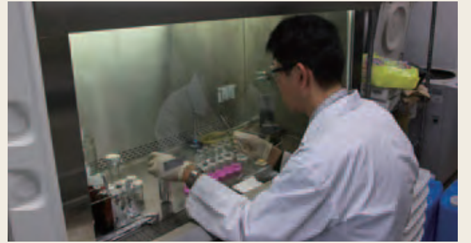
植継(細胞の増殖速度が頭打ちとなったとき、培養液を少量とって新たな培地へ移す作業)をしながら目的の微生物を増殖させる。
